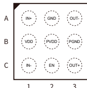
QFN1.5x1.5-9L
