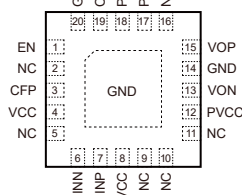
QFN3X3-20L
