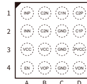
FCQFN1.6x1.6-16L
