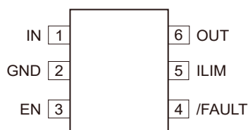
SOT23-6
