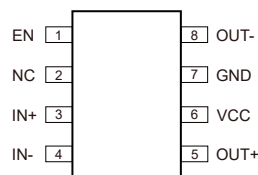
SOP8/MSOP8
