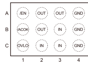
WLCSP-12L
